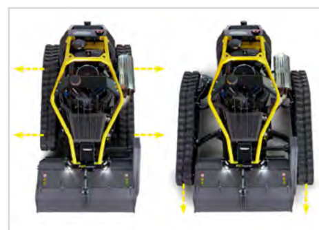
SISTEMA PATENTADO DE ELEVACIÓN con variación del centro de gravedad de la máquina
